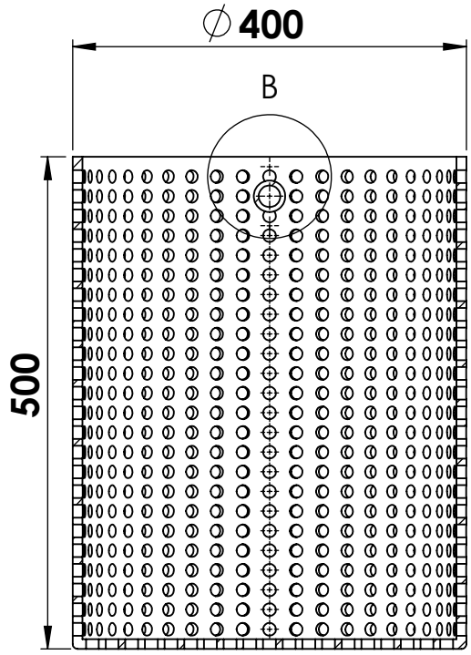
SECTION A-A SCALE 1 : 7
