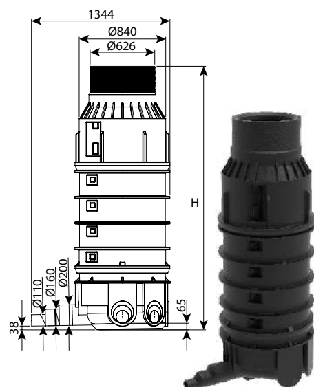
תא בקרה קומפלט ריתוך קוטר 80 מפלס 0 - 5 כניסות, מדרגות משולבות, 90°
