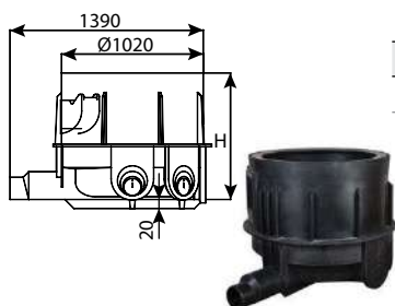
חוליית בסיס קוטר 100 - 5 כניסות קוטר 20, מדרגות אינטגרליות, מפלס 0, 45°
